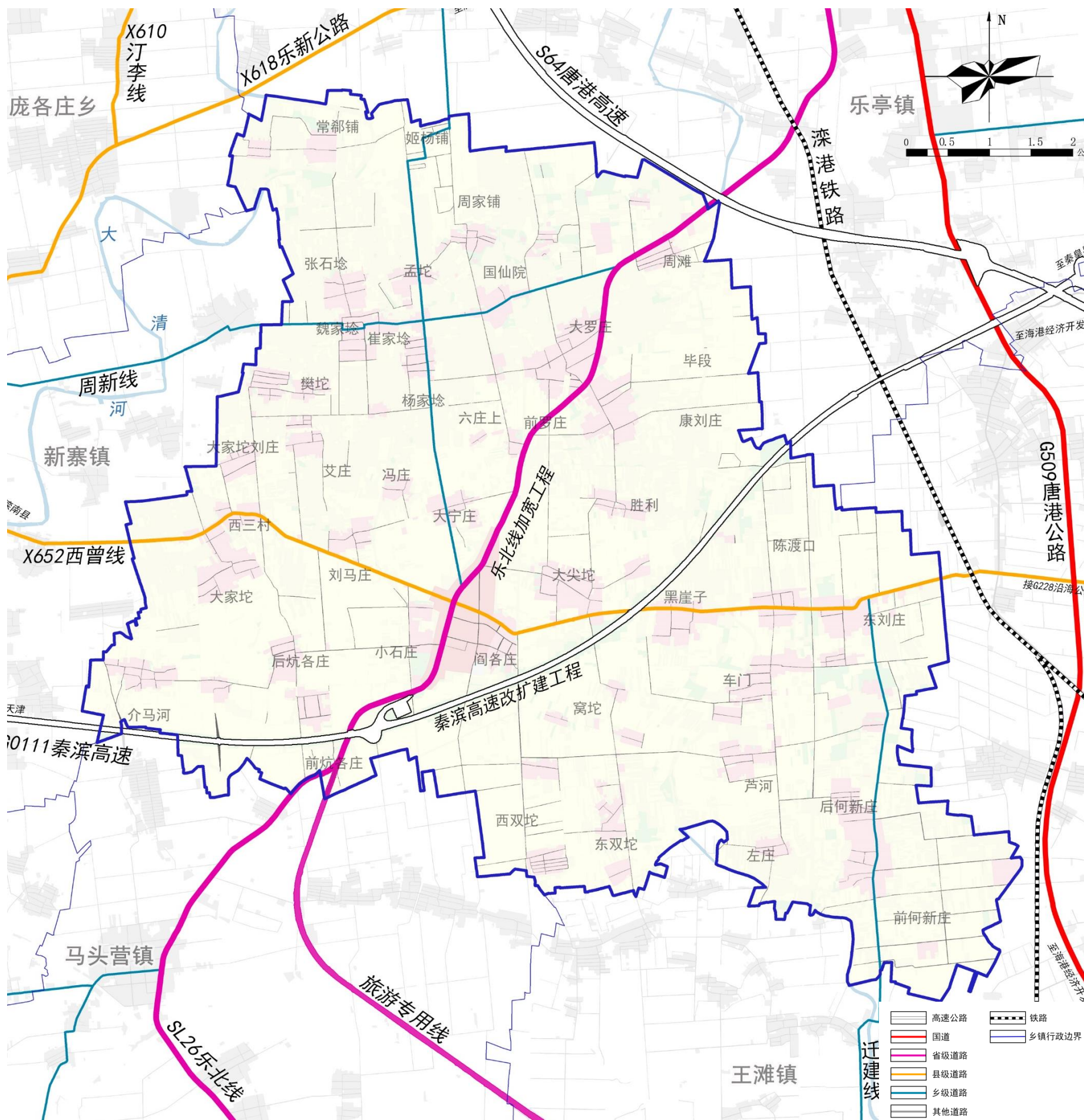
镇域综合交通规划图
