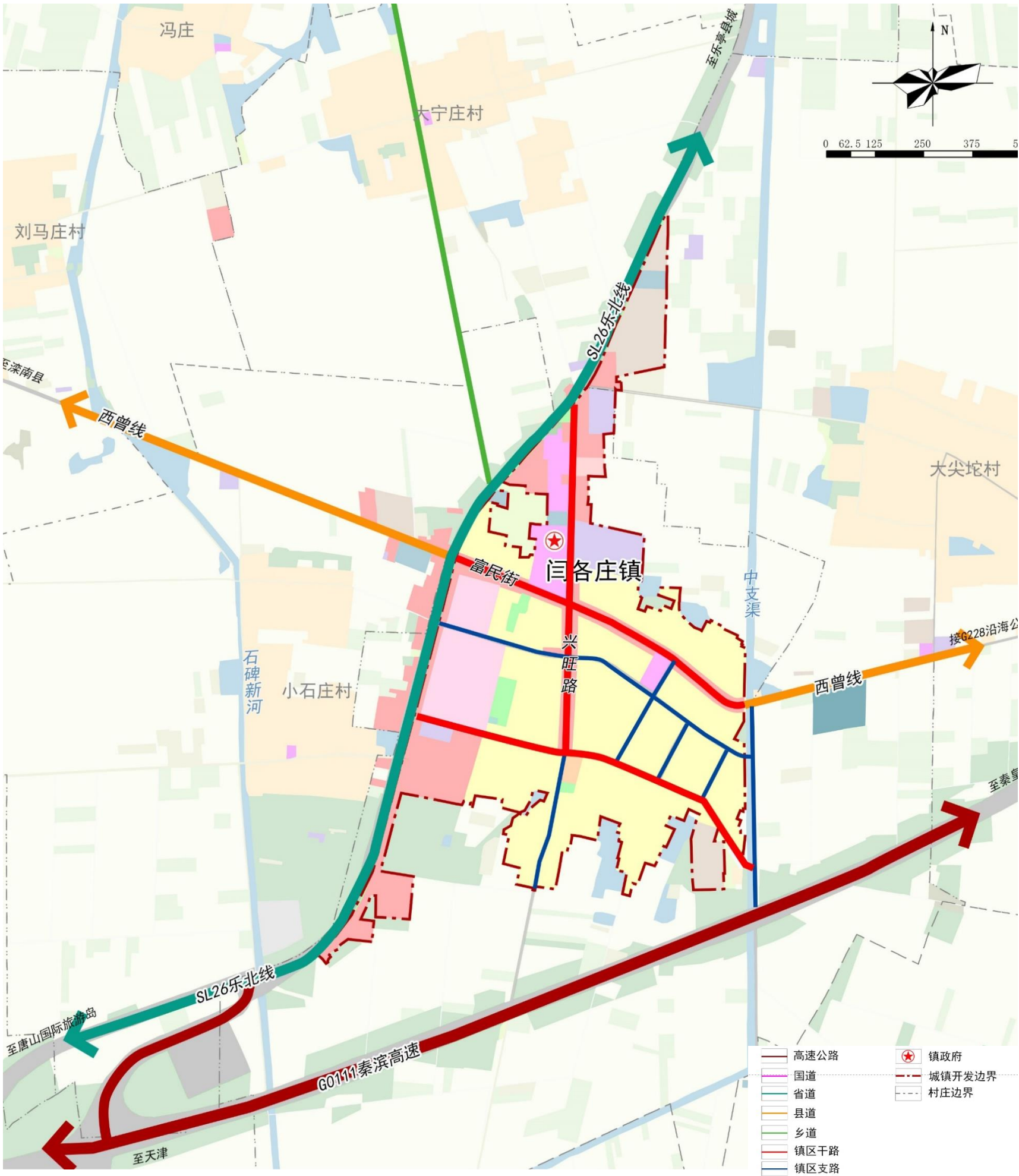
镇区道路系统规划图
