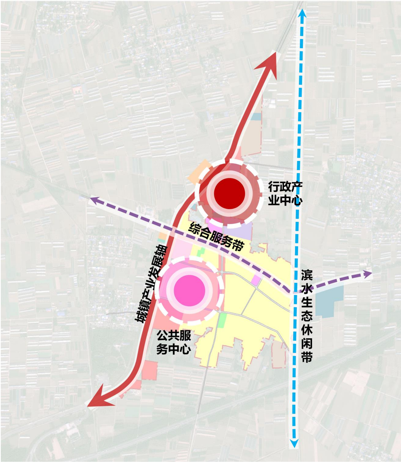
镇区空间结构规划图
