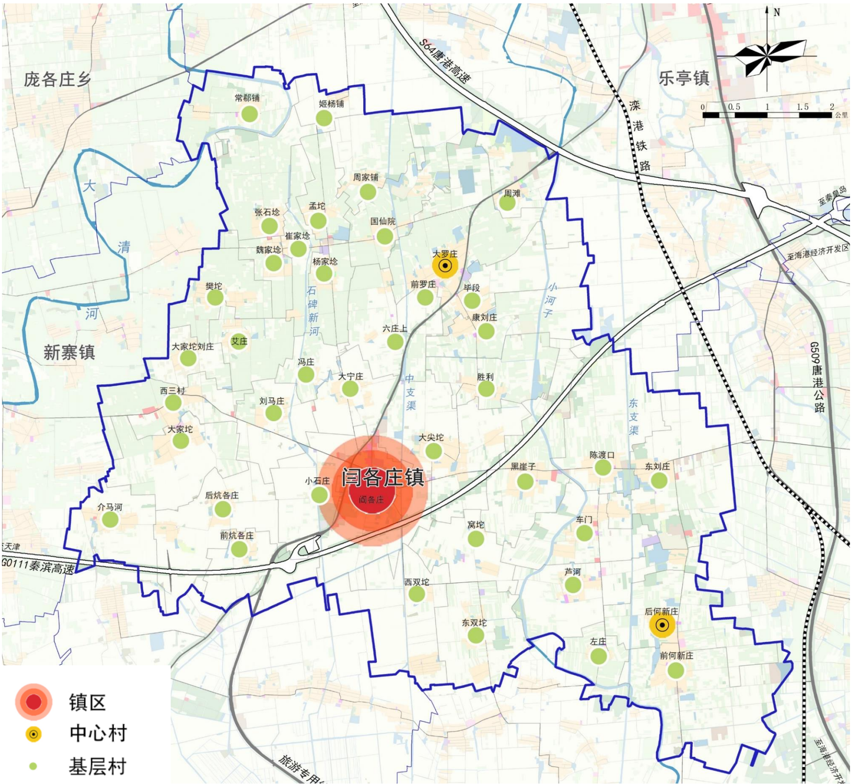
镇域村庄布点规划图
